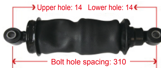
D215221440810 M3000 Rear Air Bags
